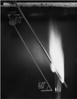
従来電線 (IV)
