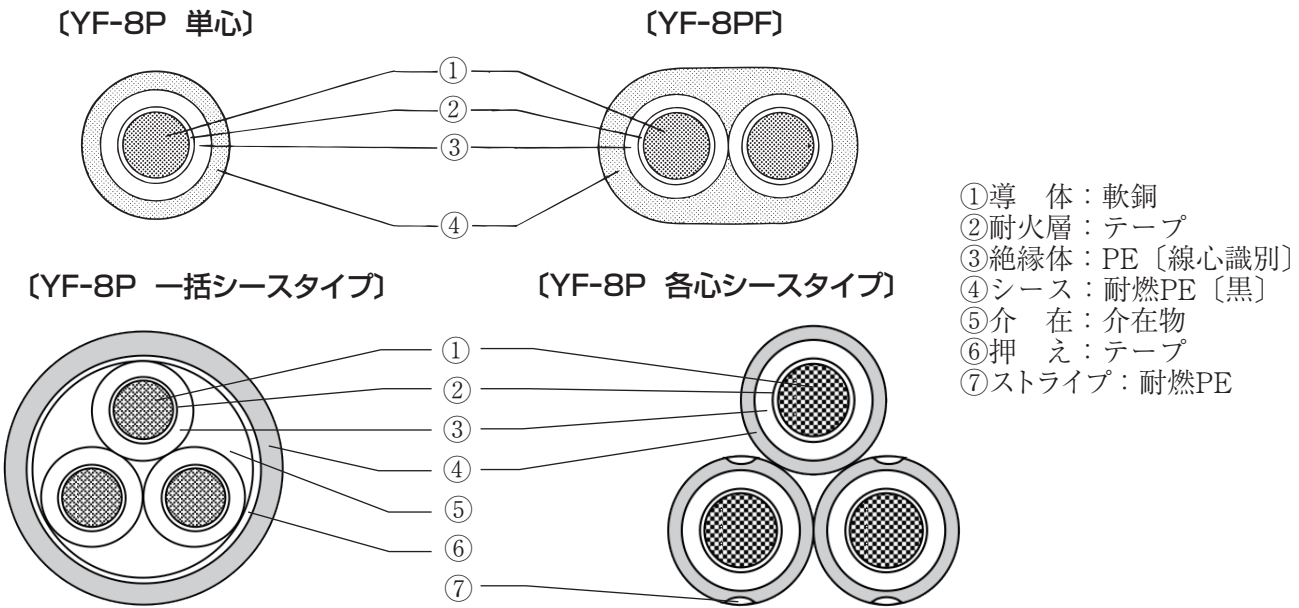
線心識別：絶縁体色〔シース表面ストライプ色〕
