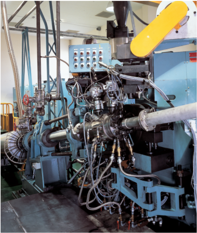
架橋ポリエチレン絶縁押出工程（沼津）
