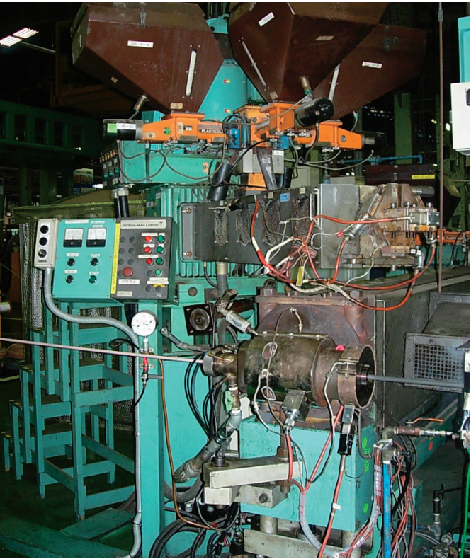
ビニルシース押出工程（沼津）
