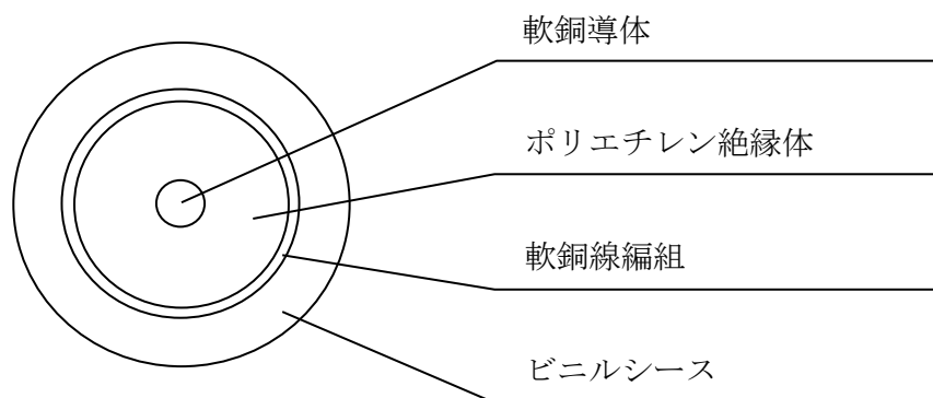
断 面 図
