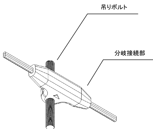
例)直接吊りボルトに取付け
