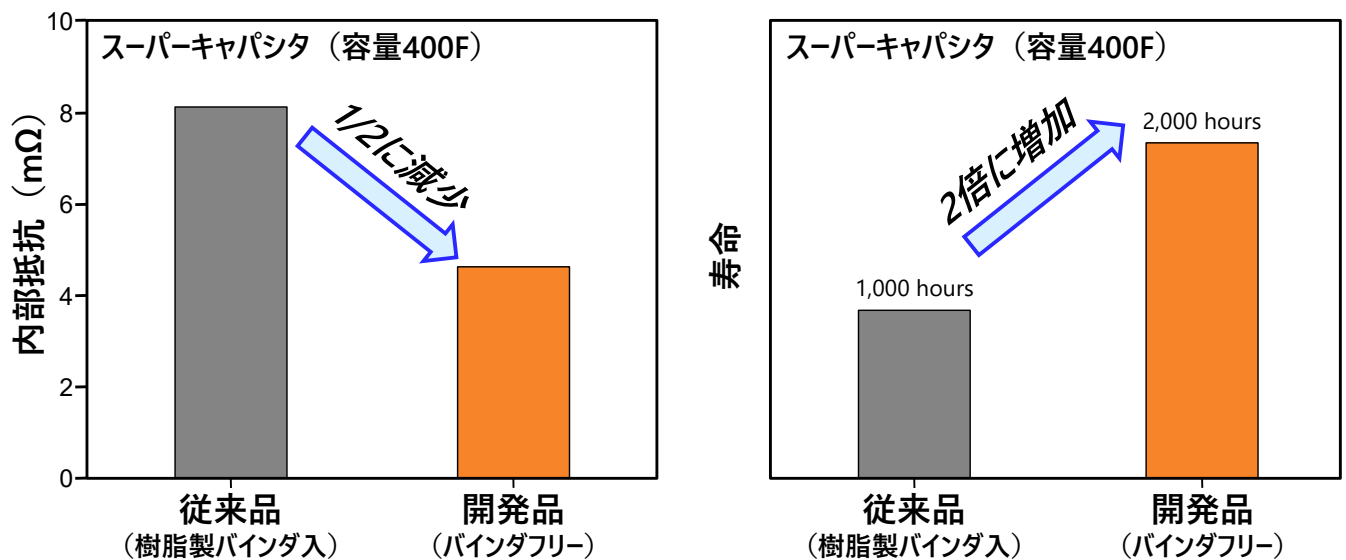
図 6 : 従来の電極とバインダフリー電極の内部抵抗と寿命比較
