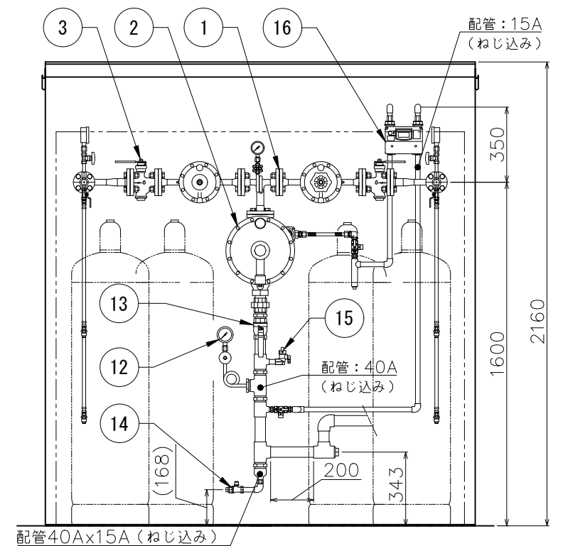
B-B (正面図)
