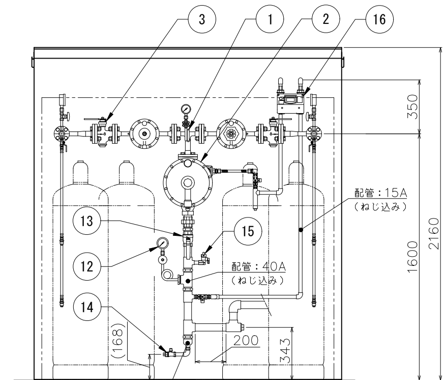
B-B (正面図)
