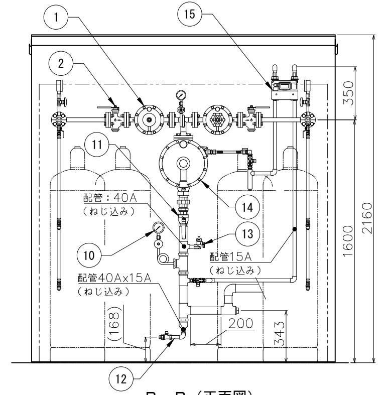
B-B (正面図)
