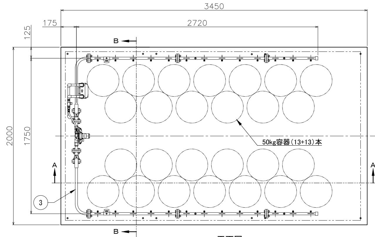
平面図
