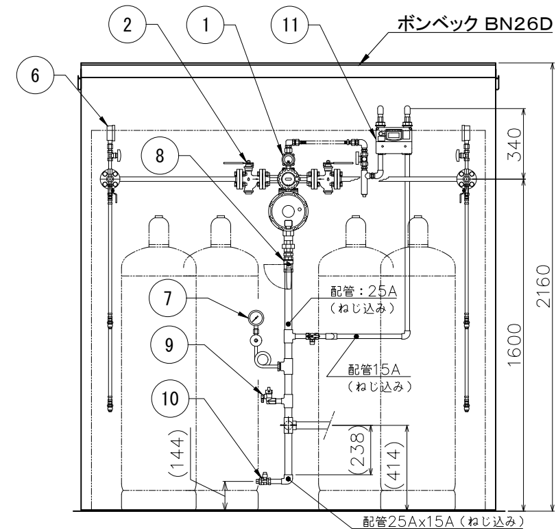
B-B (正面図)
