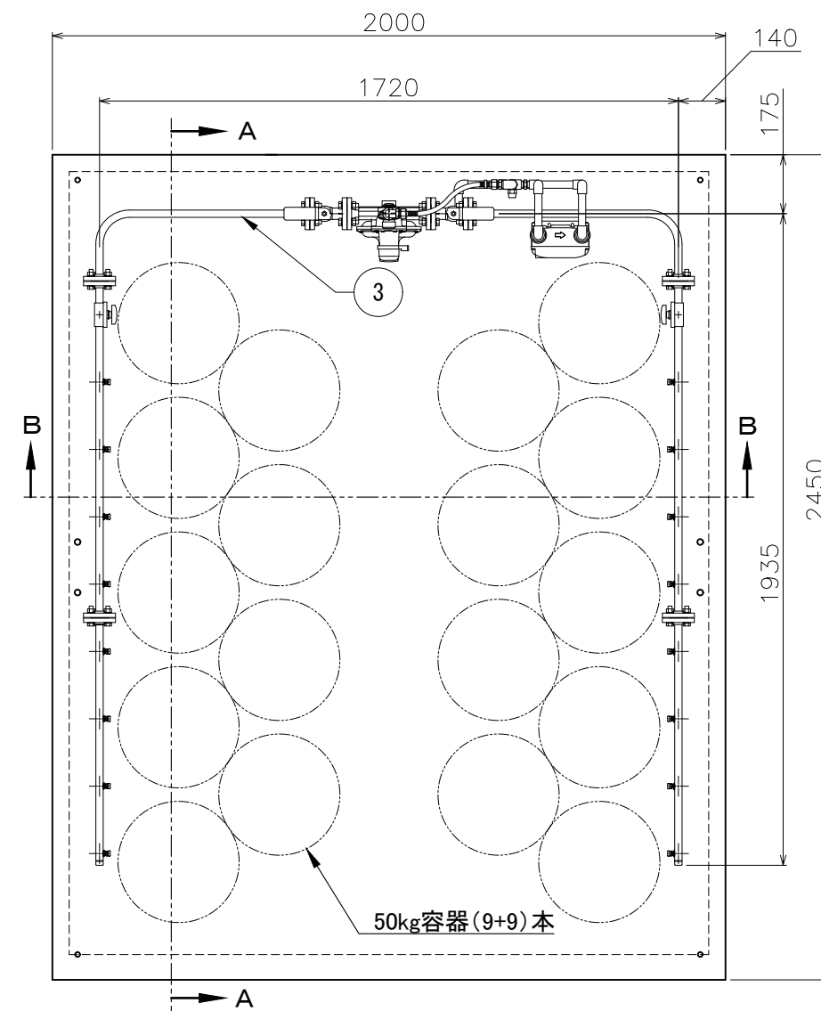
平面図
