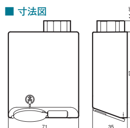
■ 寸法図
