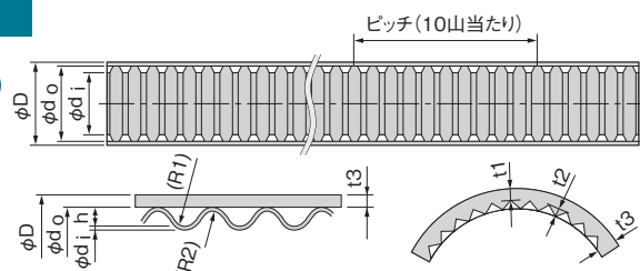
構造
