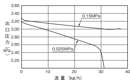
RL30 II B (P.49)
