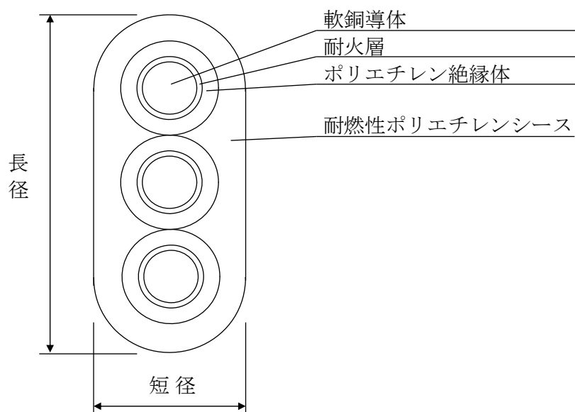
断面図
