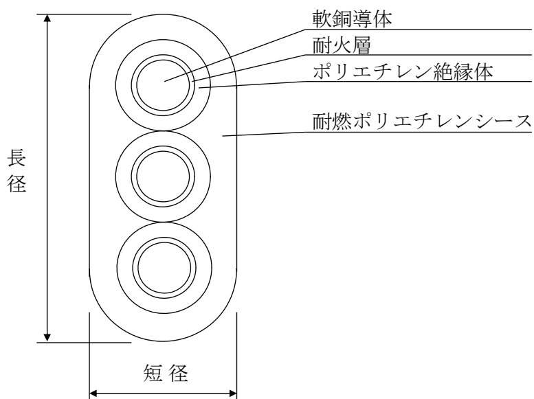
断面図
