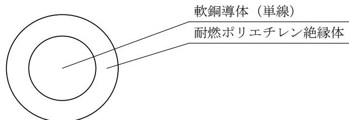
断面図 (単線)
