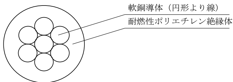
断面図 (より線)
