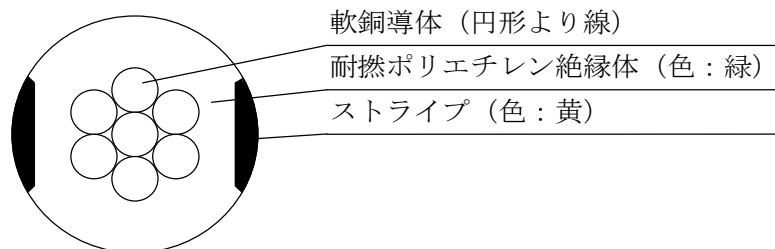
断 面 図
