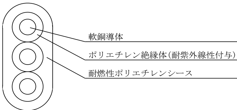
断 面 図
