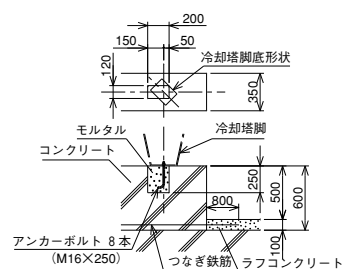
基礎参考図
