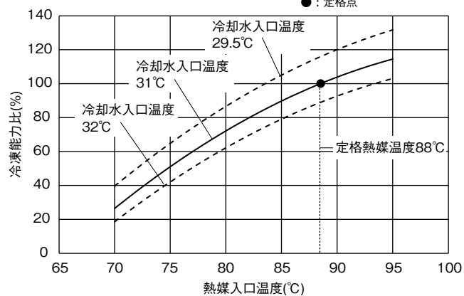
熱媒入口温度特性 (冷凍時)
