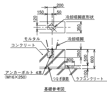
基礎参考図
