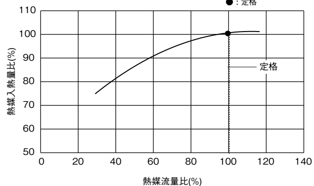
熱媒流量特性 (冷凍時)
