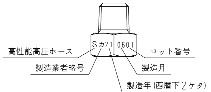
レーザー印字の内容 (A矢視)
