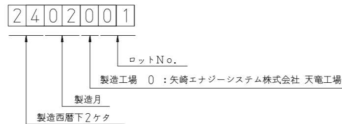
刻印詳細図
