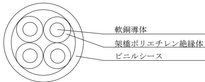
断 面 図
