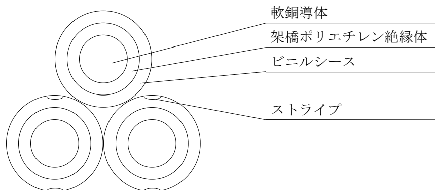
断 面 図
