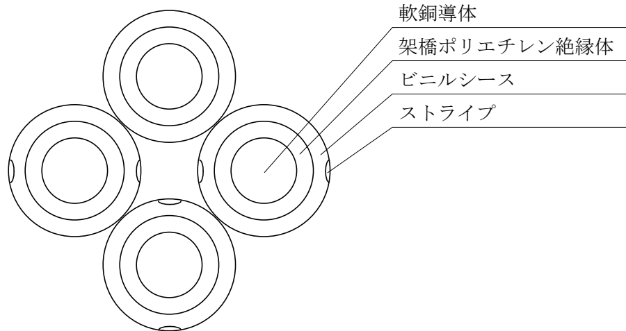
断 面 図
