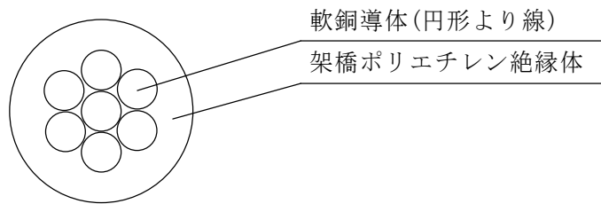
断 面 図
