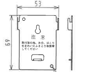
取付板 (1コ)
