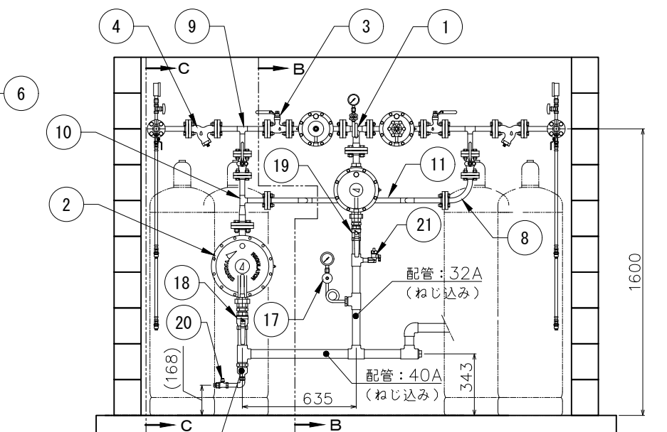
配管40Ax15A (ねじ込み) A-A (正面図)
