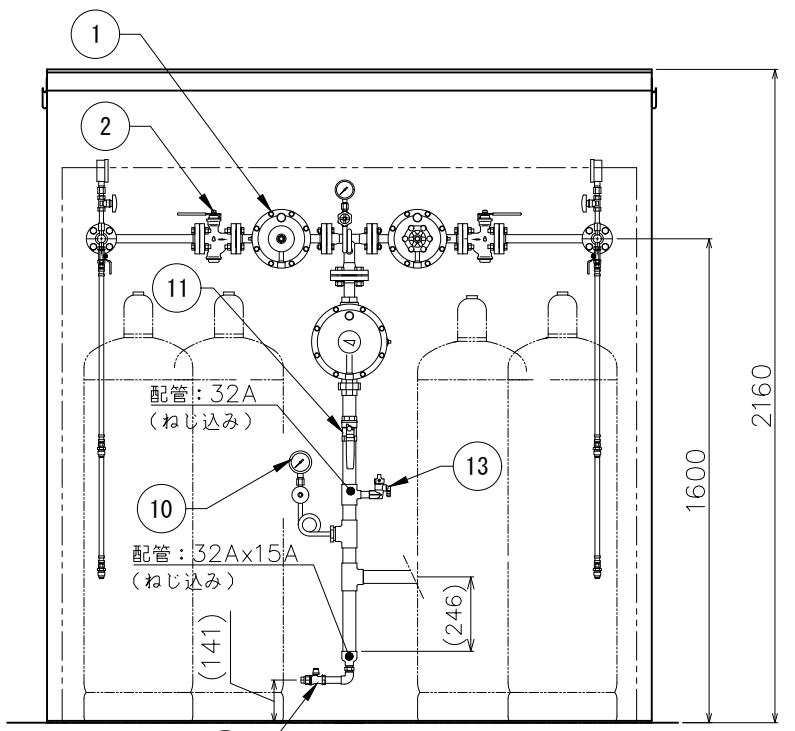
B-B (正面図)
