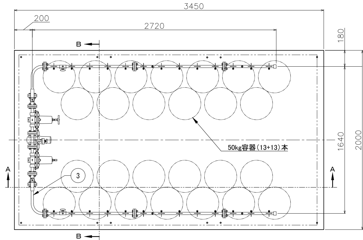
平面図
