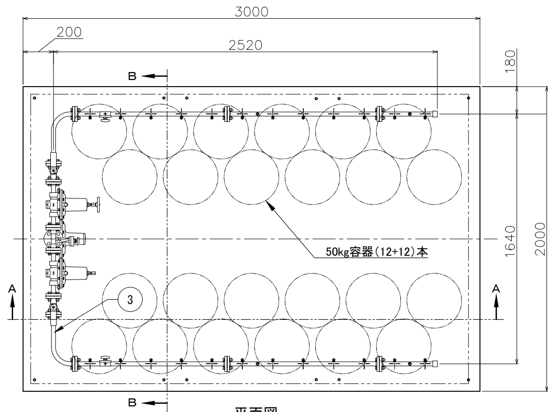
平面図
