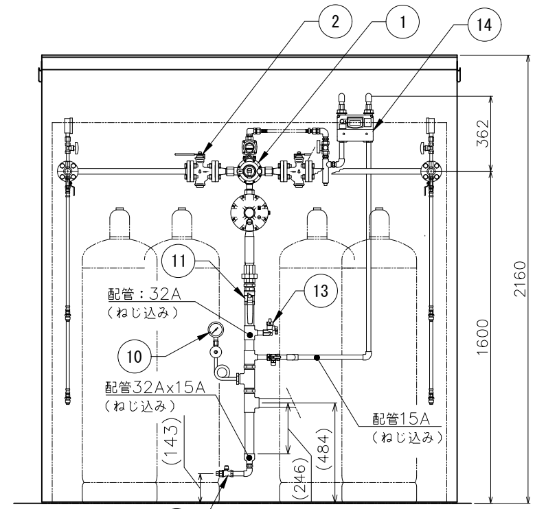
B-B (正面図)
