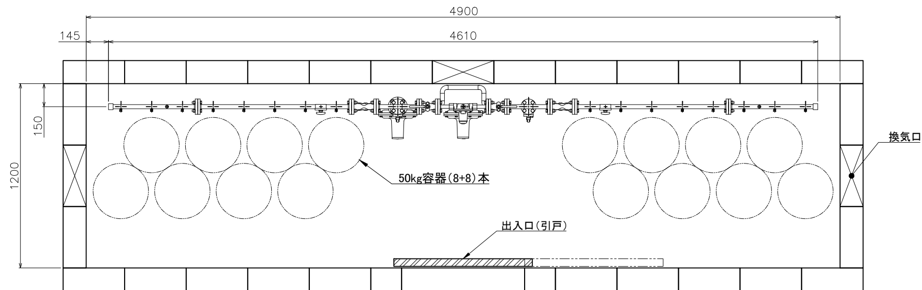
平面図
