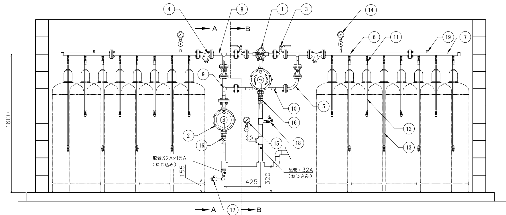
正面図
