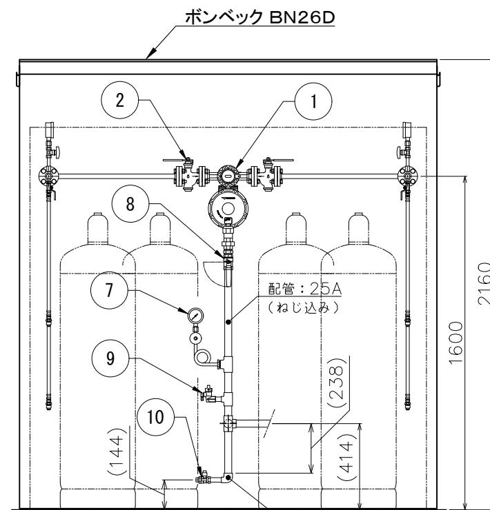
B-B (正面図)
