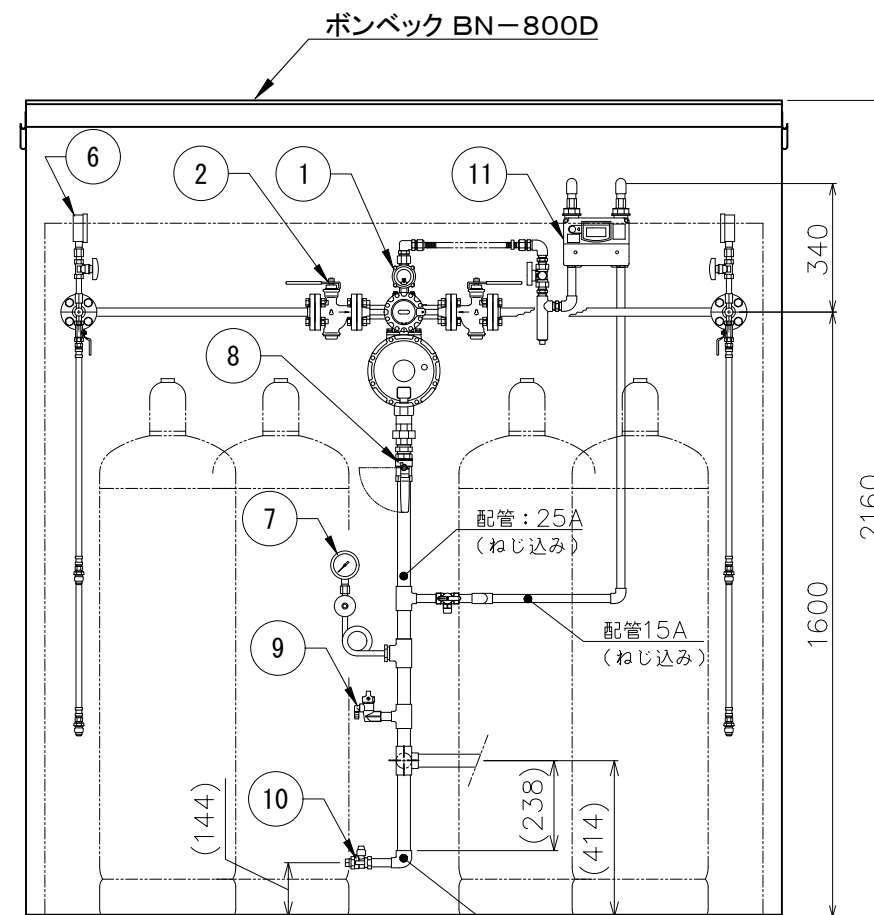
B-B (正面図)
