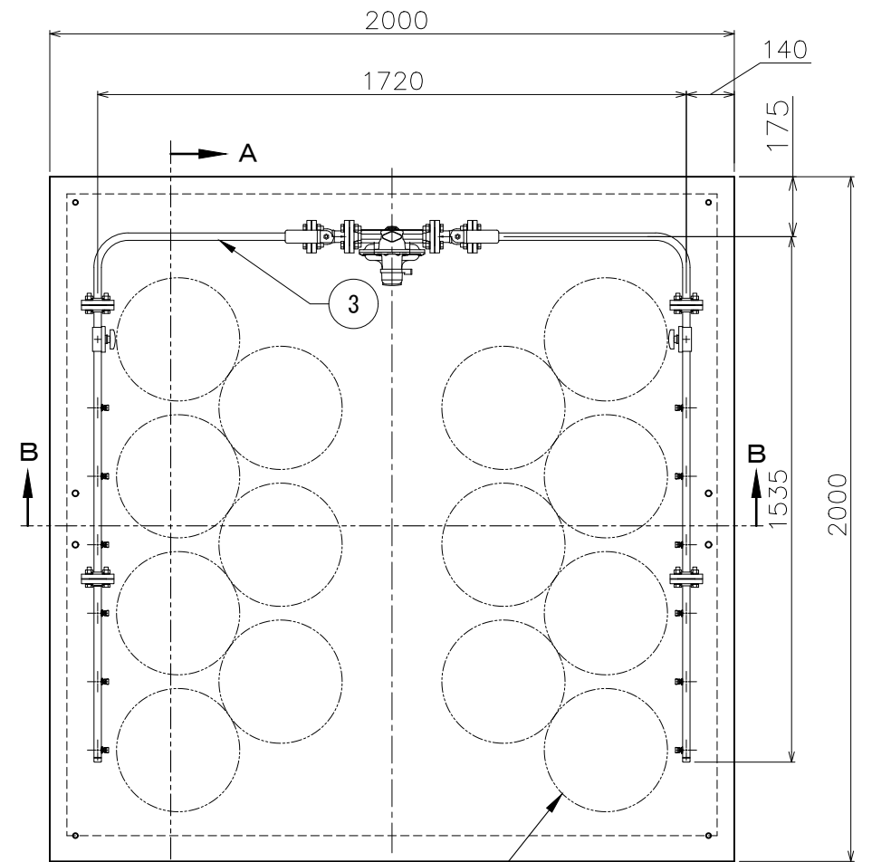
平面図
