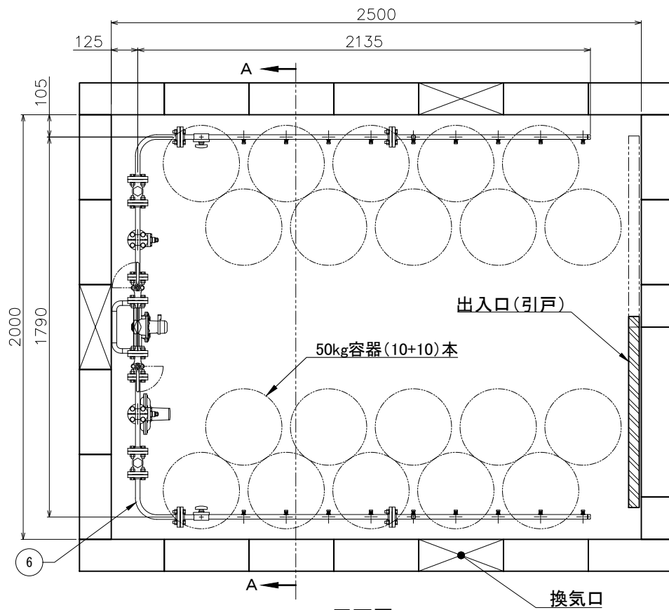
平面図
