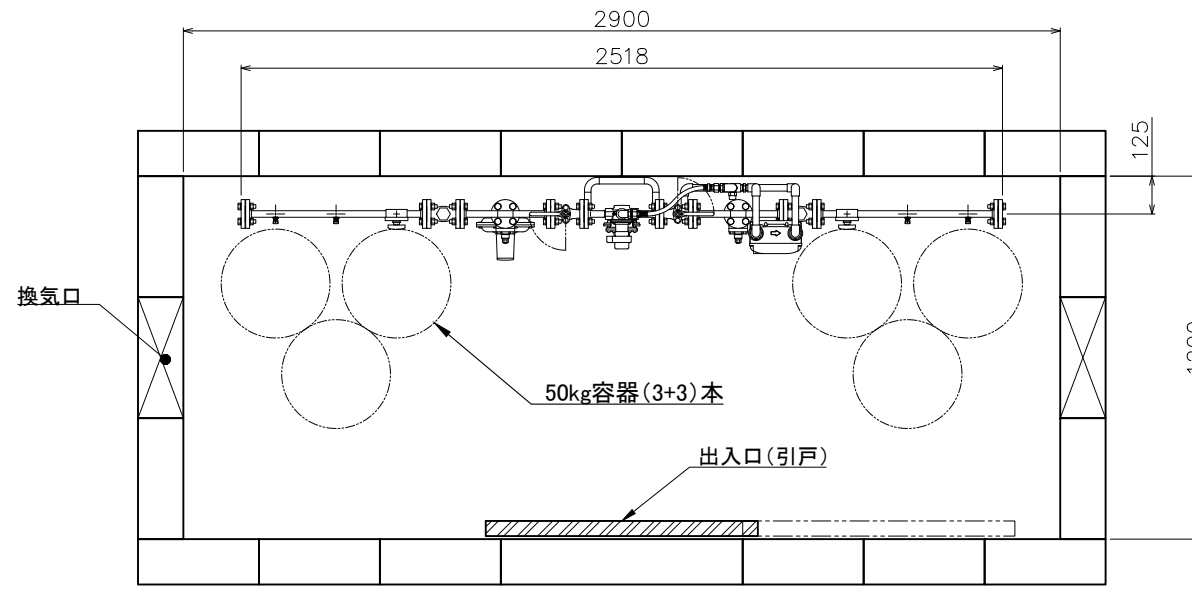
平面図
