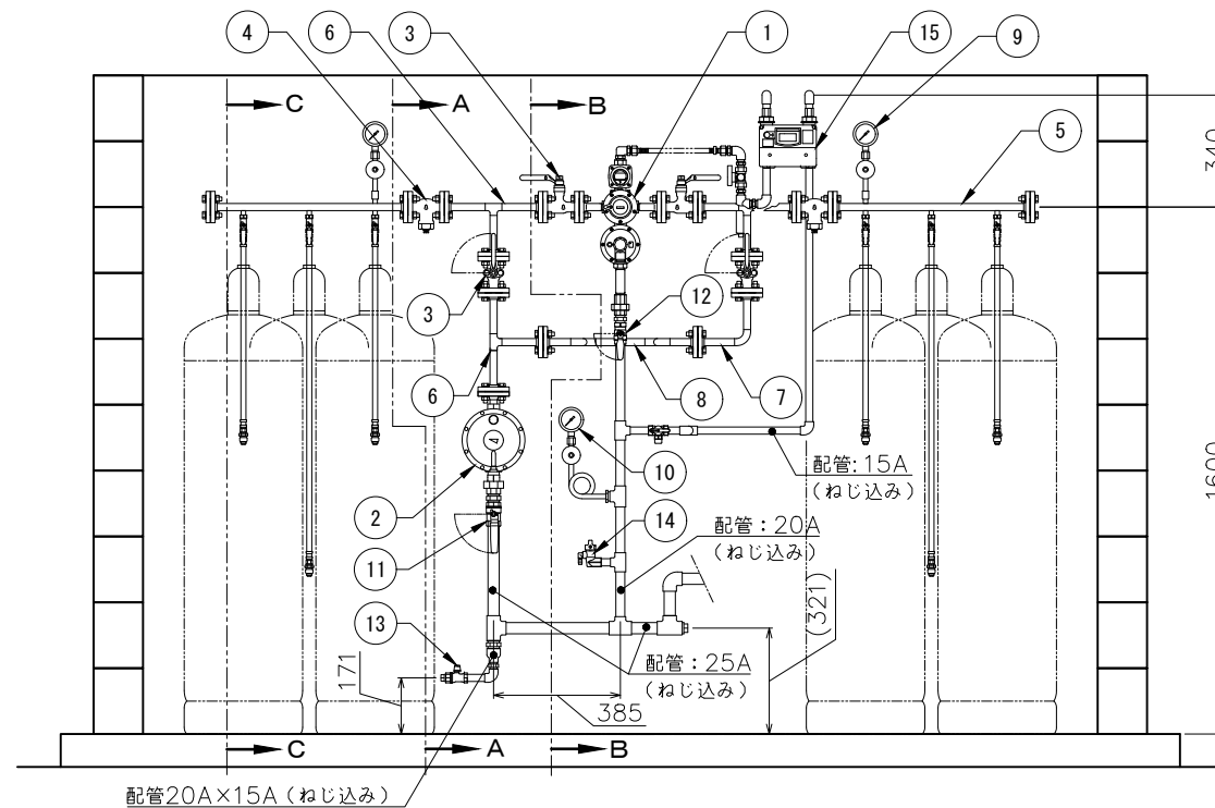
正面図
