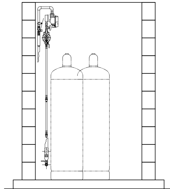
C-C (左側面図)
