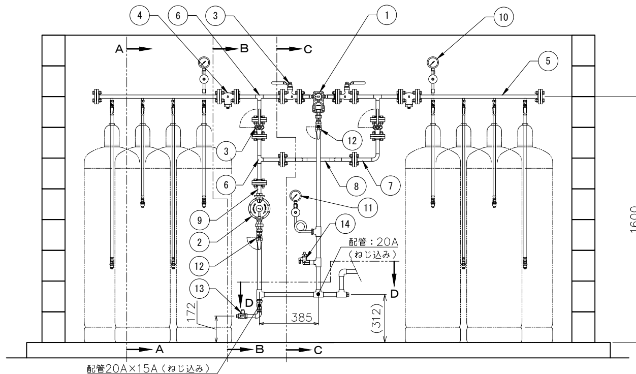
正面図
