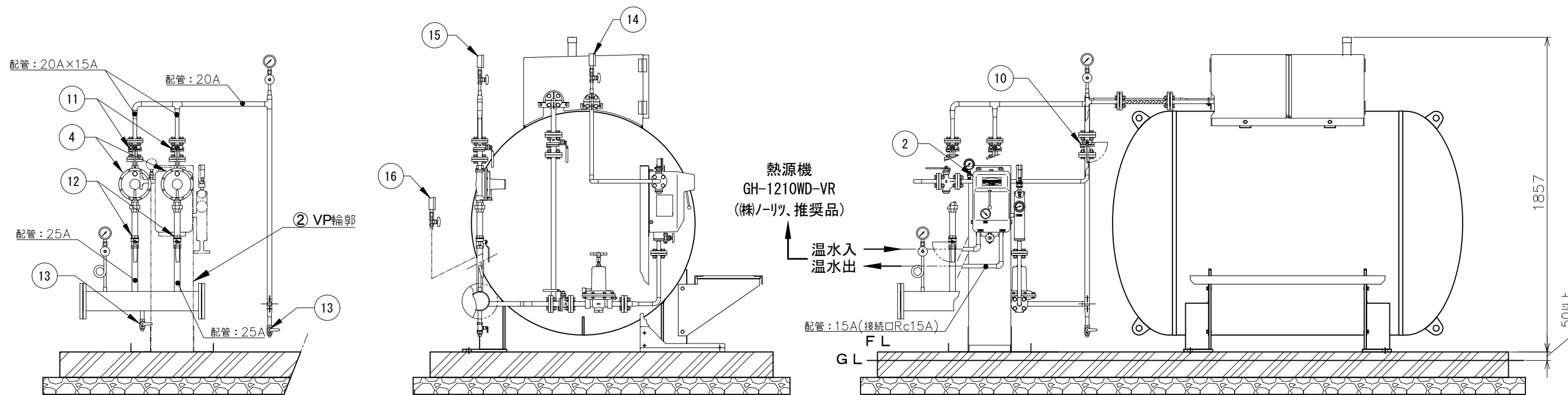
A-A (二段二次調整器部配管)
