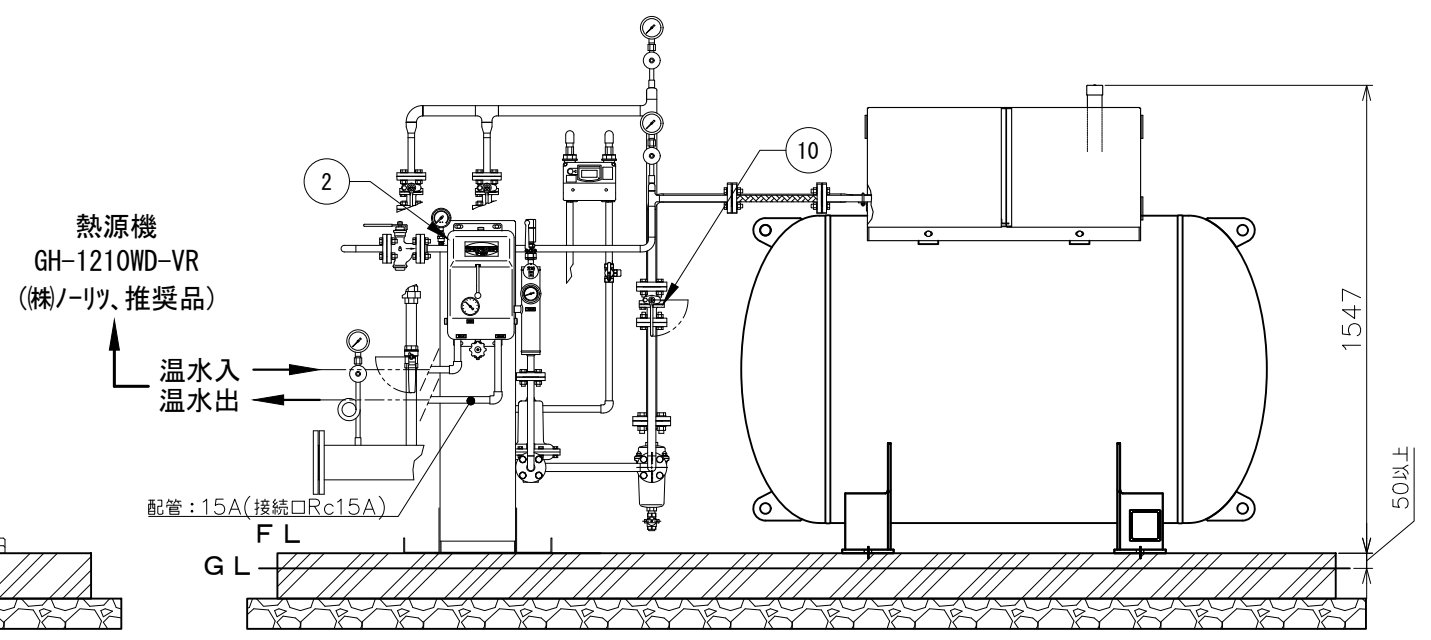
正面図
