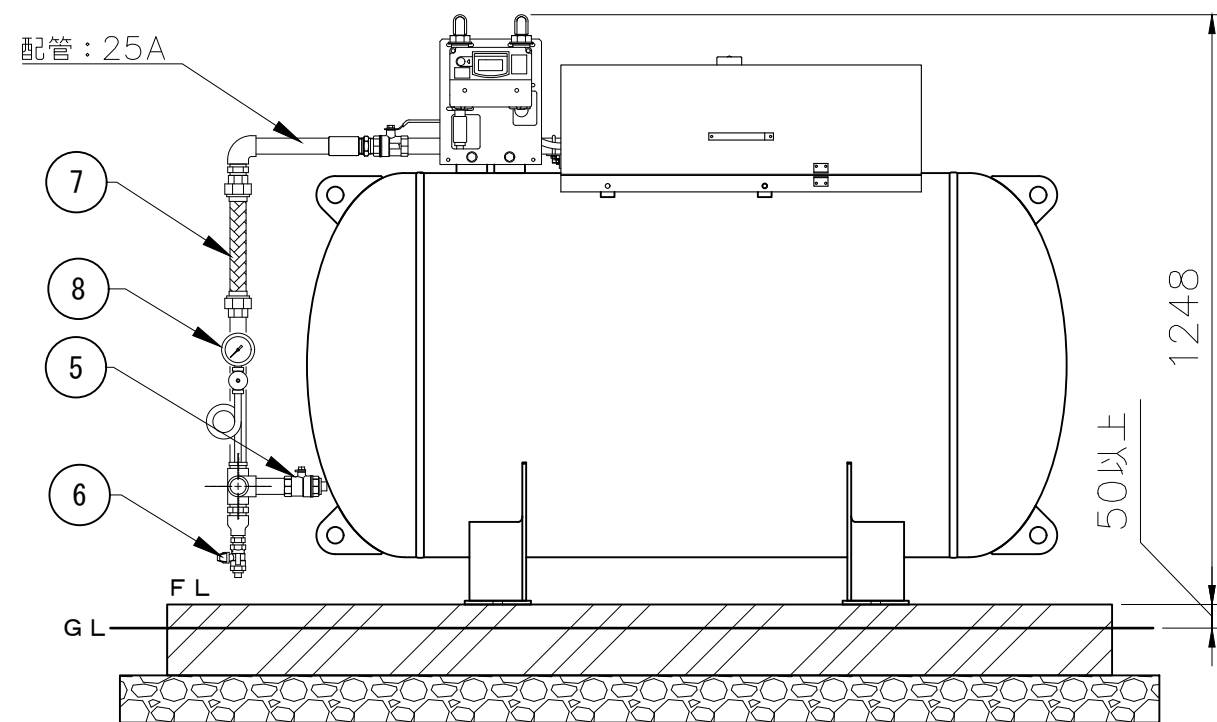
正面図
